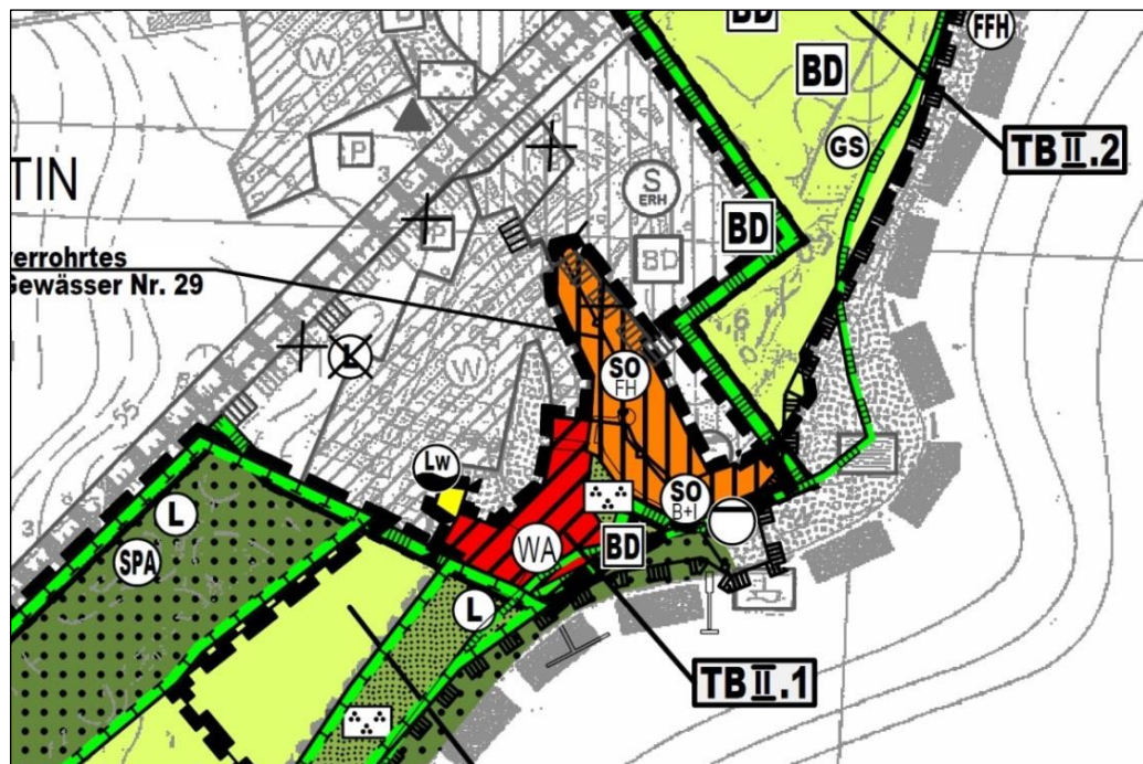
Abb. 3: Darstellungen der 2. Änderung des Flächennutzungsplanes für den Bereich der 2. Änderung des Bebauungsplanes Nr. 14A
